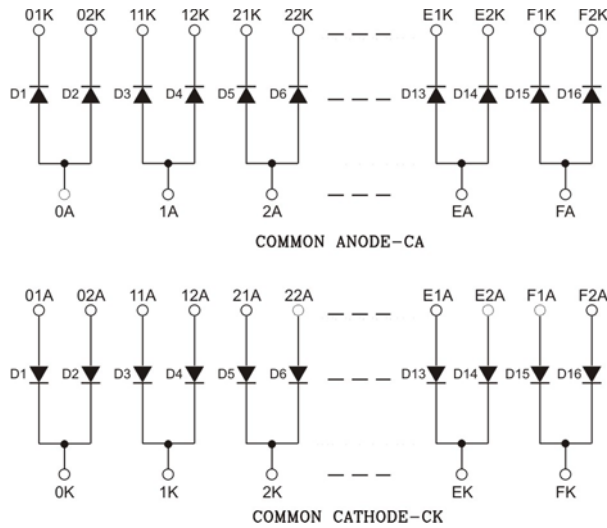
Diode Module Schematic
